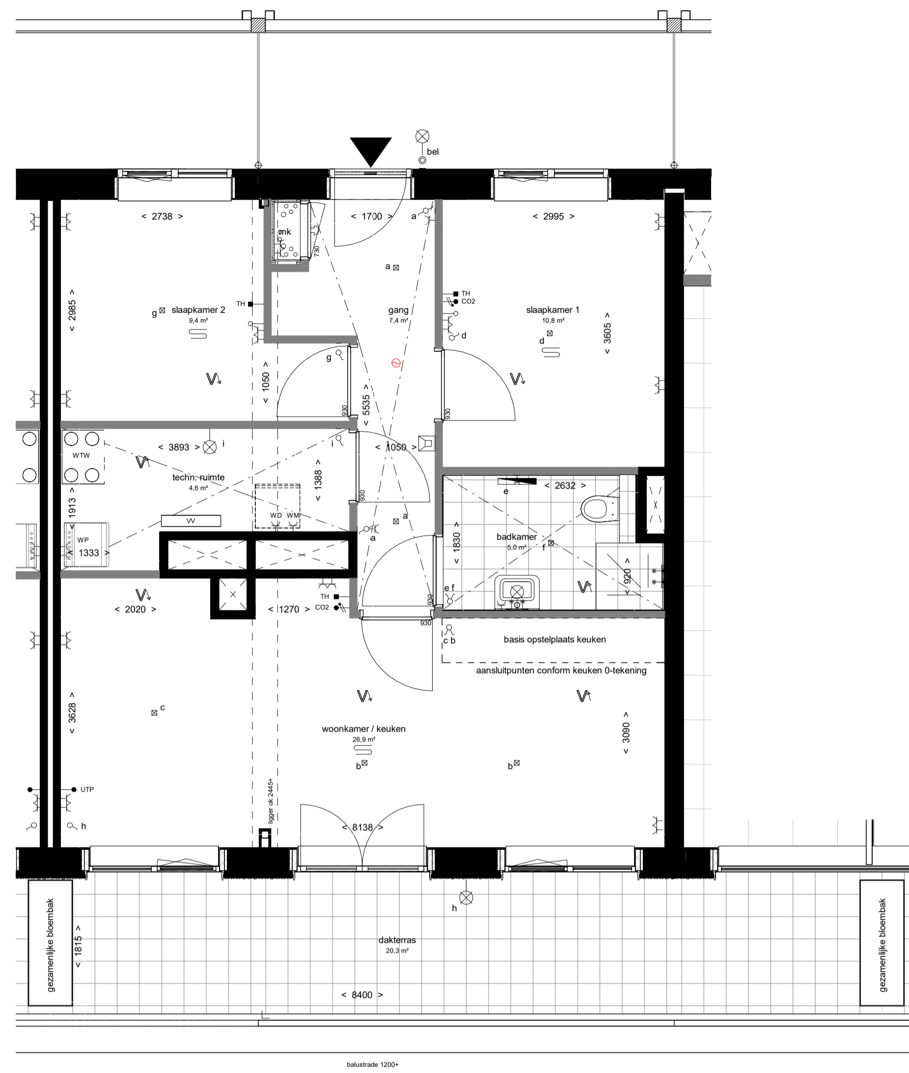
5e verdieping - type I2 - BNR 5.02
